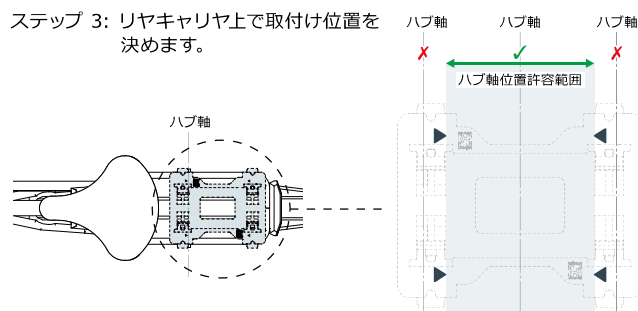
キャリヤ取付金具
